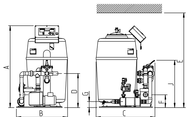
Abb. 3 Maßzeichnung Filteranlage GENO-mat® F 600 HK; DS
