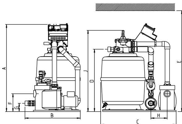
Abb. 2 Maßzeichnung Filteranlage GENO-mat® F 500 HK; WS
